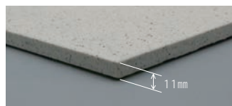
曲げ破壊荷重 (N) 約 1,200N
