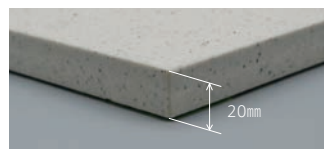
曲げ破壊荷重 (N) 約 4,800N
