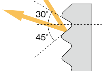
クールアイランドタイルの 反射特性
